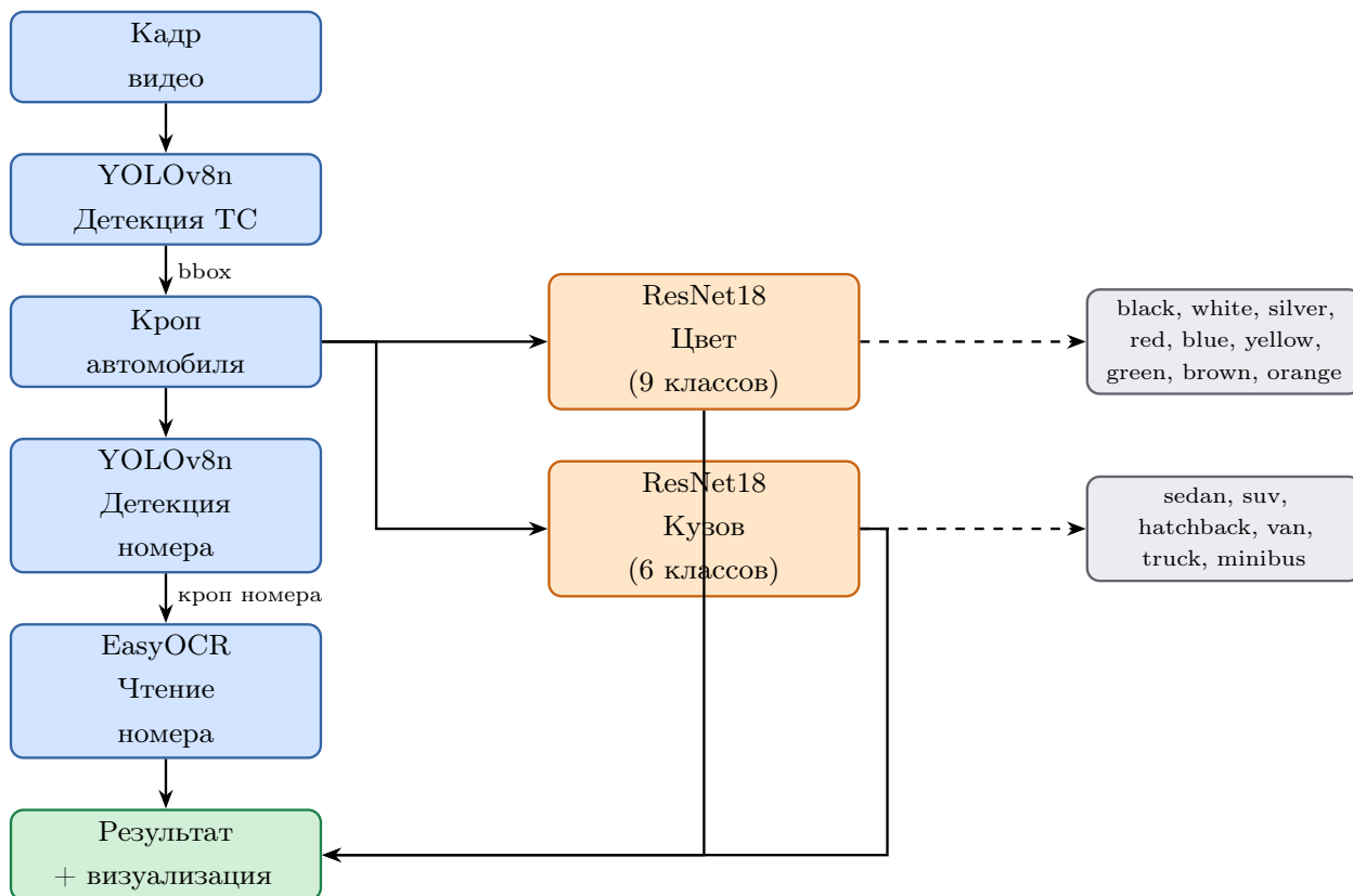
Figure 2.1: Схема конвейера обработки видеокadra
