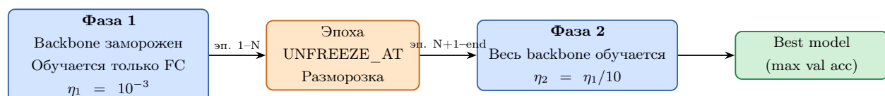
Figure 2.6: Стратегия двухфазного дообучения ResNet18
